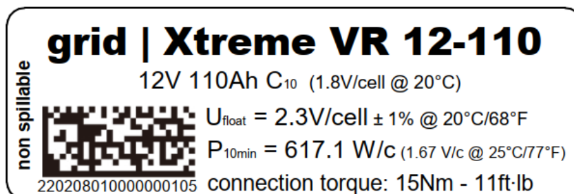
Abbildung 3-1 - Typenschild
