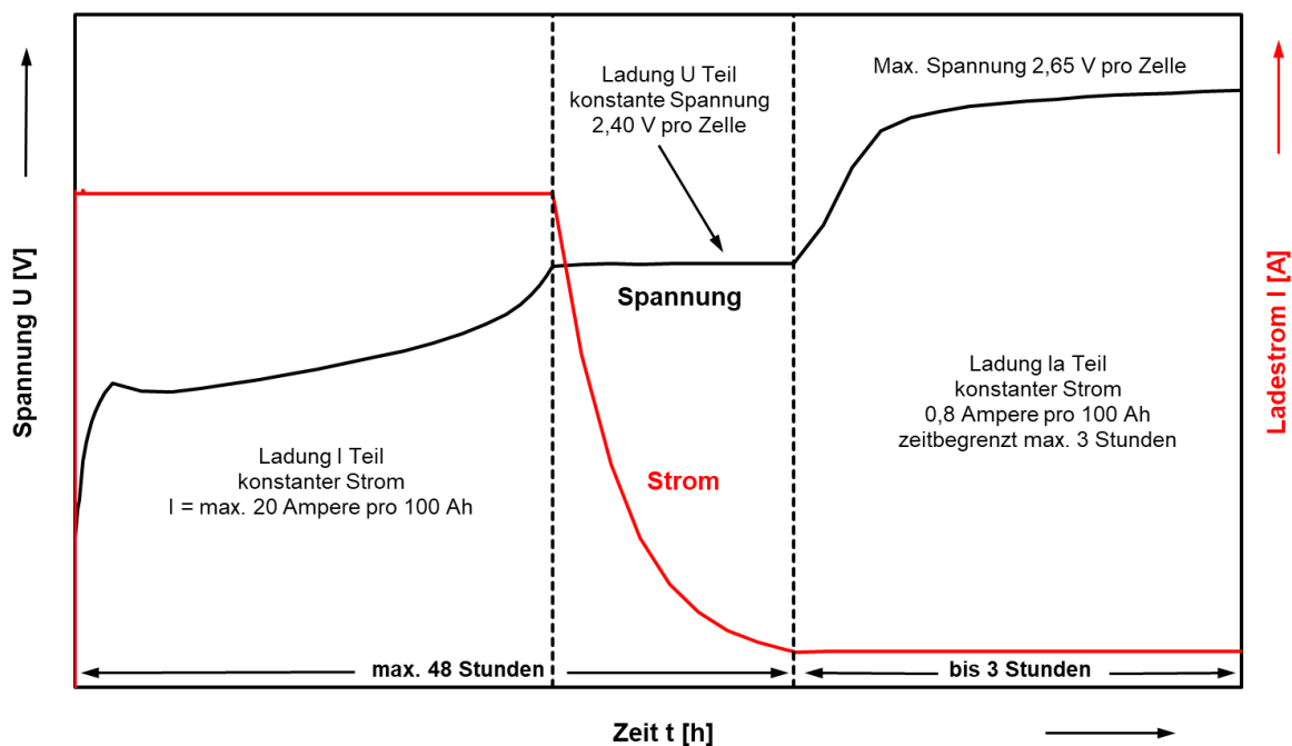
Abbildung 8-2 - Kennlinie IUIa
