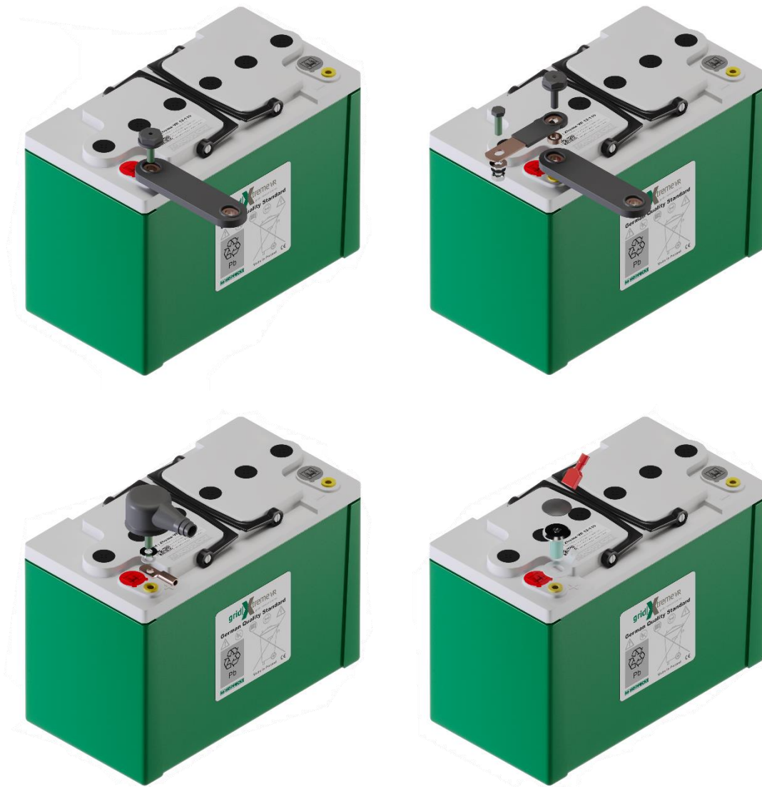
Abbildung 6.6.6-1 - Polanschlussmöglichkeiten für Zellenverbindung (starre und flexible Verbinder), Mittenabgriff, Gruppen- und Endverbindung und Zellenverbindung mit Batterieüberwachungssystem.
