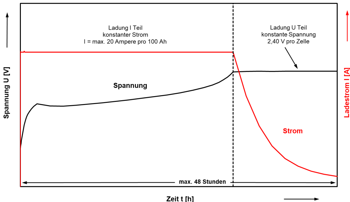
Abbildung 8-1 - Kennlinie IU
