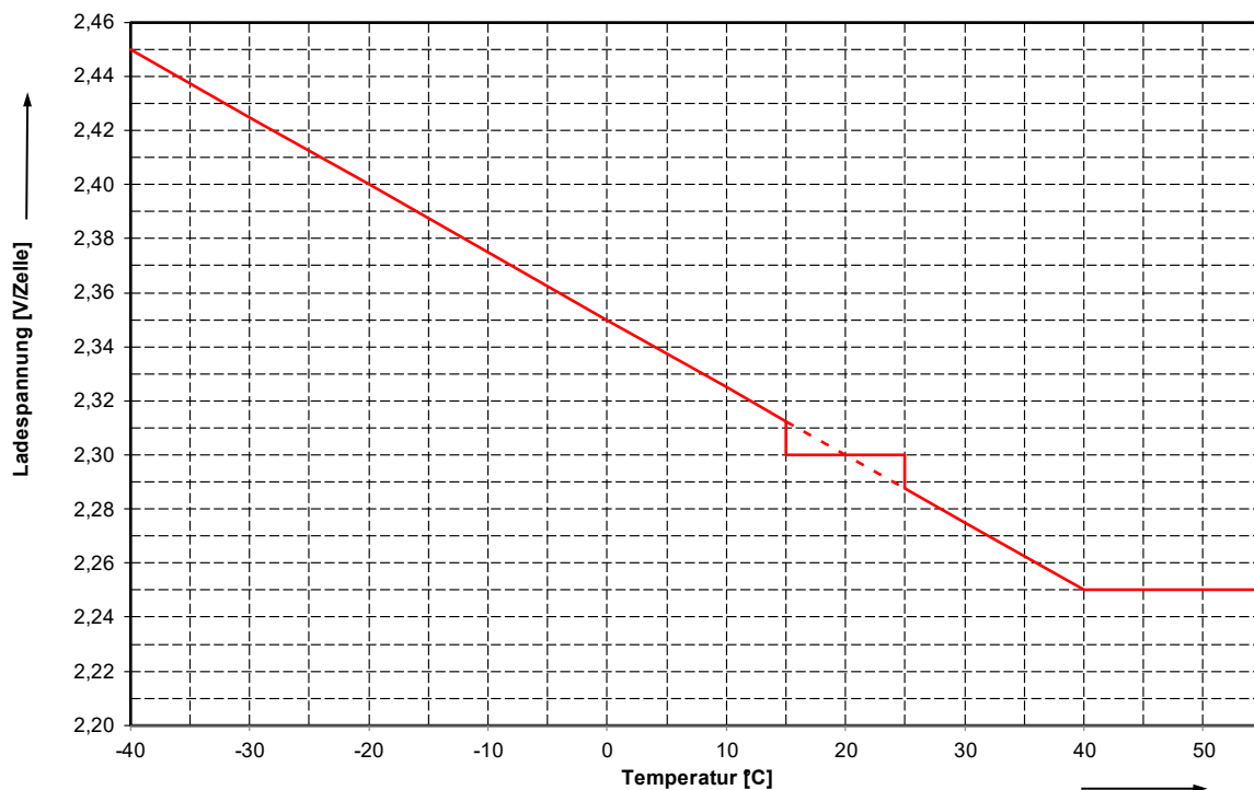
Abbildung 7.2.2-1 - Temperaturabhängige Anpassung der Ladeerhaltungsspannung für grid | Xtreme VR mit einer Ladeerhaltungsspannung von 2,30 V/Zelle bei T_{\text{nenn}}
